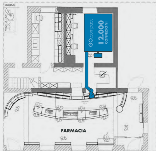
SOLUZIONE DI INSTALLAZIONE 1
